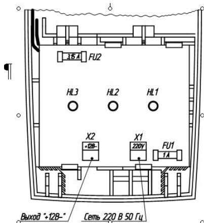
Рисунок 4- Обозначение клемм и места установки вставок плавких (исп. 01, исп.02)
