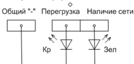
Рисунок 1 – Схема подключения источника к ВУОС
